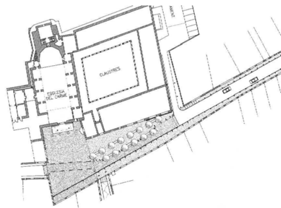
Planta general àmbit actuació urbanització Plaça del Carme. OLOT
